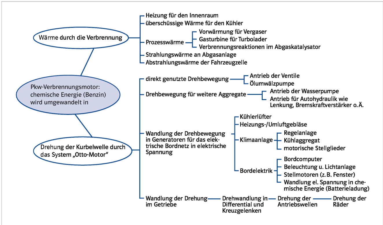
1 Einige Energieumwandlungen in unserem Beispiel-Pkw
