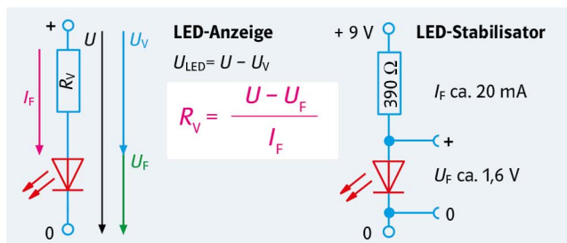
3 Leuchtdiode mit Vorwiderstand
